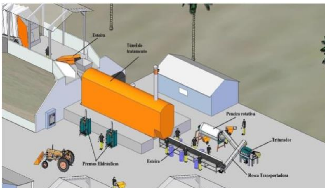
FIGURA 4: INFRA-ESTRUTURA DE UMA CENTRAL DE TRIAGEM E COMPOSTAGEM
