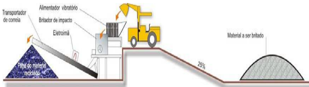
Figura: Representação Esquemática da Estação de reciclagem
